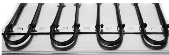
Монтажная лента, подклеенная специальной самоклеящейся лентой RT-L500-S-AL – длина рейки - 50 см
