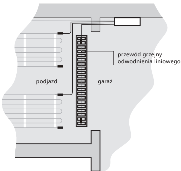
Ogrzewanie odwodnienia liniowego
