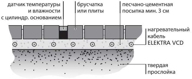
Поперечное сечение тротуара или подъездных путей, изготовленных из плит или брусчатки.
